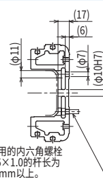
截面C-C
